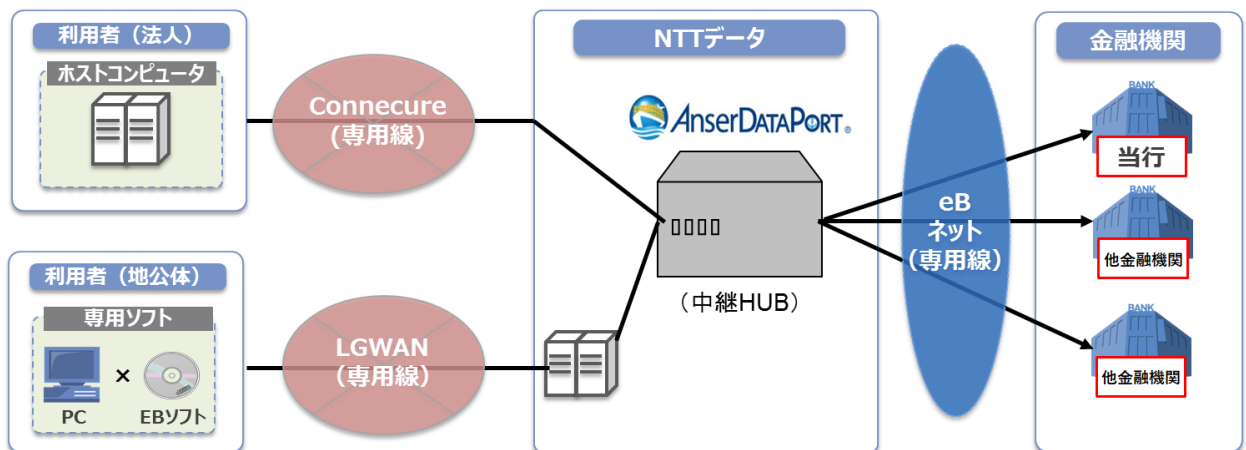
【AnserDATAPORT のイメージ図】
